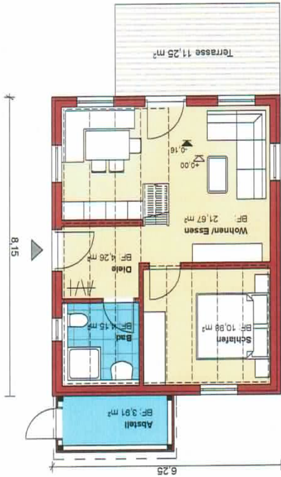
Grundriss Erdgeschoss
